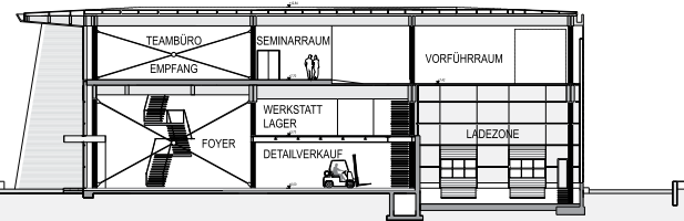
SCHNITT AA
