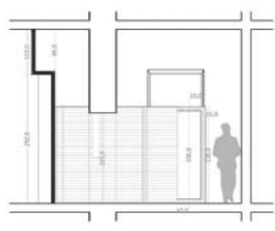
Sezione BB
